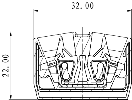
剖面 A-A
