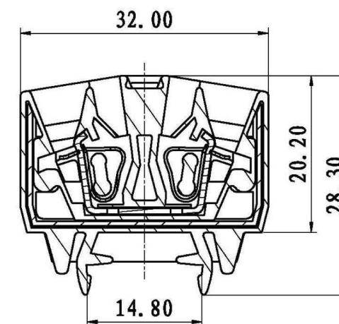
剖面 A-A
